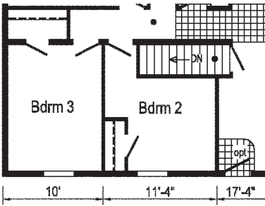
Optional Stairwell w/ Optional Bedroom 4
